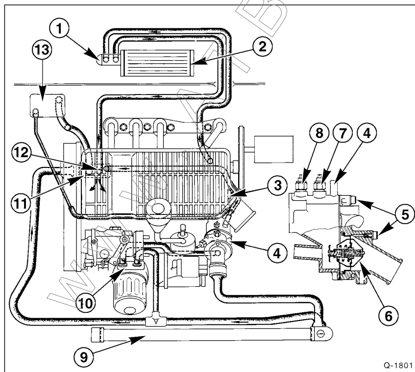
Kühlkreislauf, 1,9-l-PEUGEOT/CITROËN-Motor
